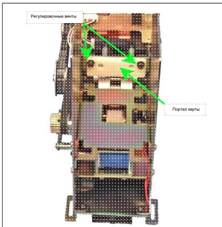
Рисунок 17 – Детали, используемые для регулировки зазора в соответствии
