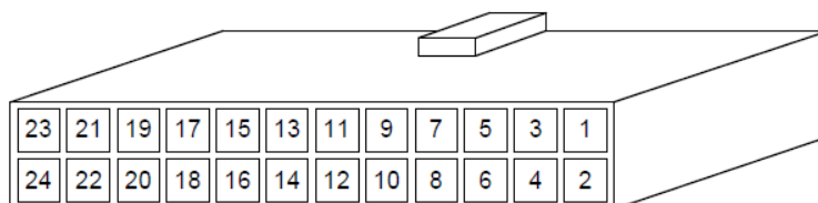
Рисунок 1 – Корпус сопрягающего соединителя интерфейса управления
