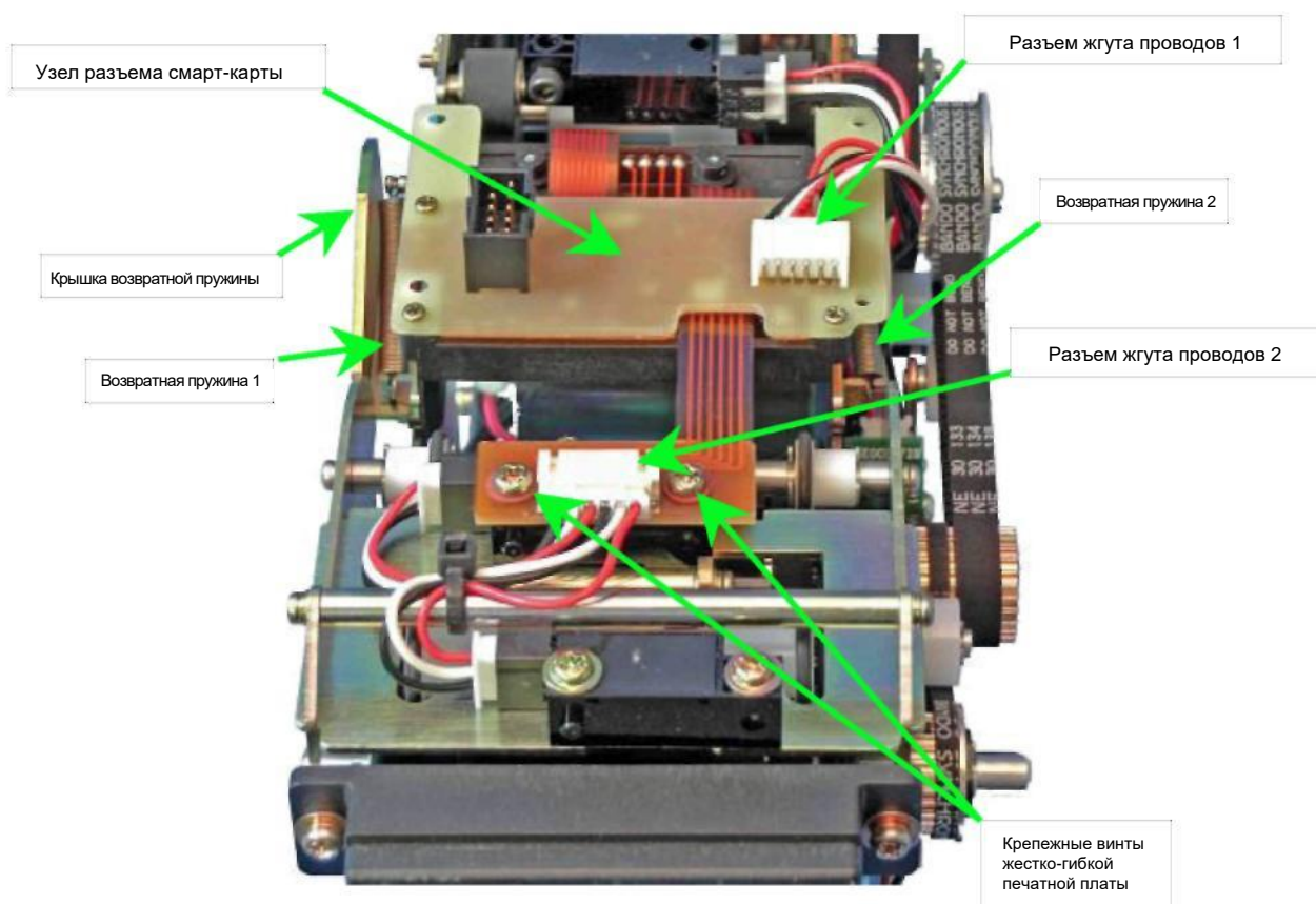
Рисунок 20а – Снятие деталей узла разъема смарт-карт
