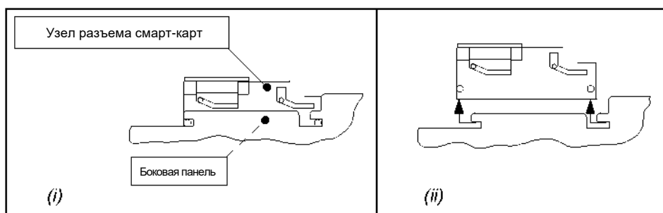
Рисунок 21 – Снятие деталей узла разъема смарт-карт
