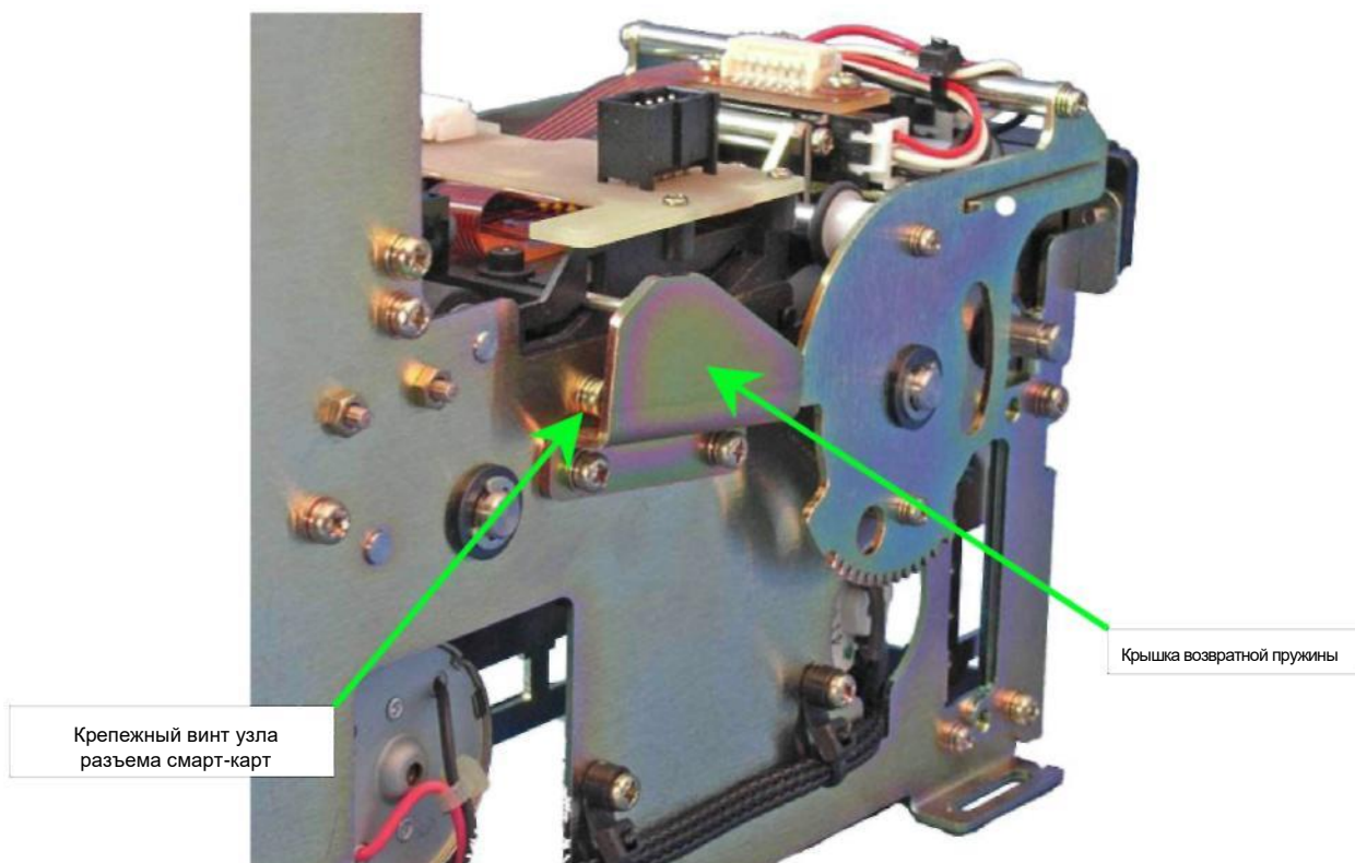
Рисунок 20b – Снятие деталей узла разъема смарт-карт
