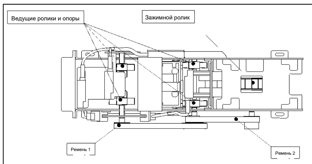
Рисунок 16 – Устройство SCD-1000, вид сверху
