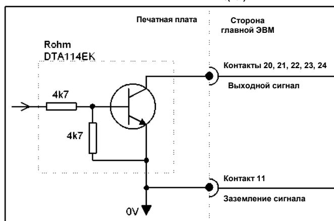
Рисунок 3 – Цепь выходного сигнала
