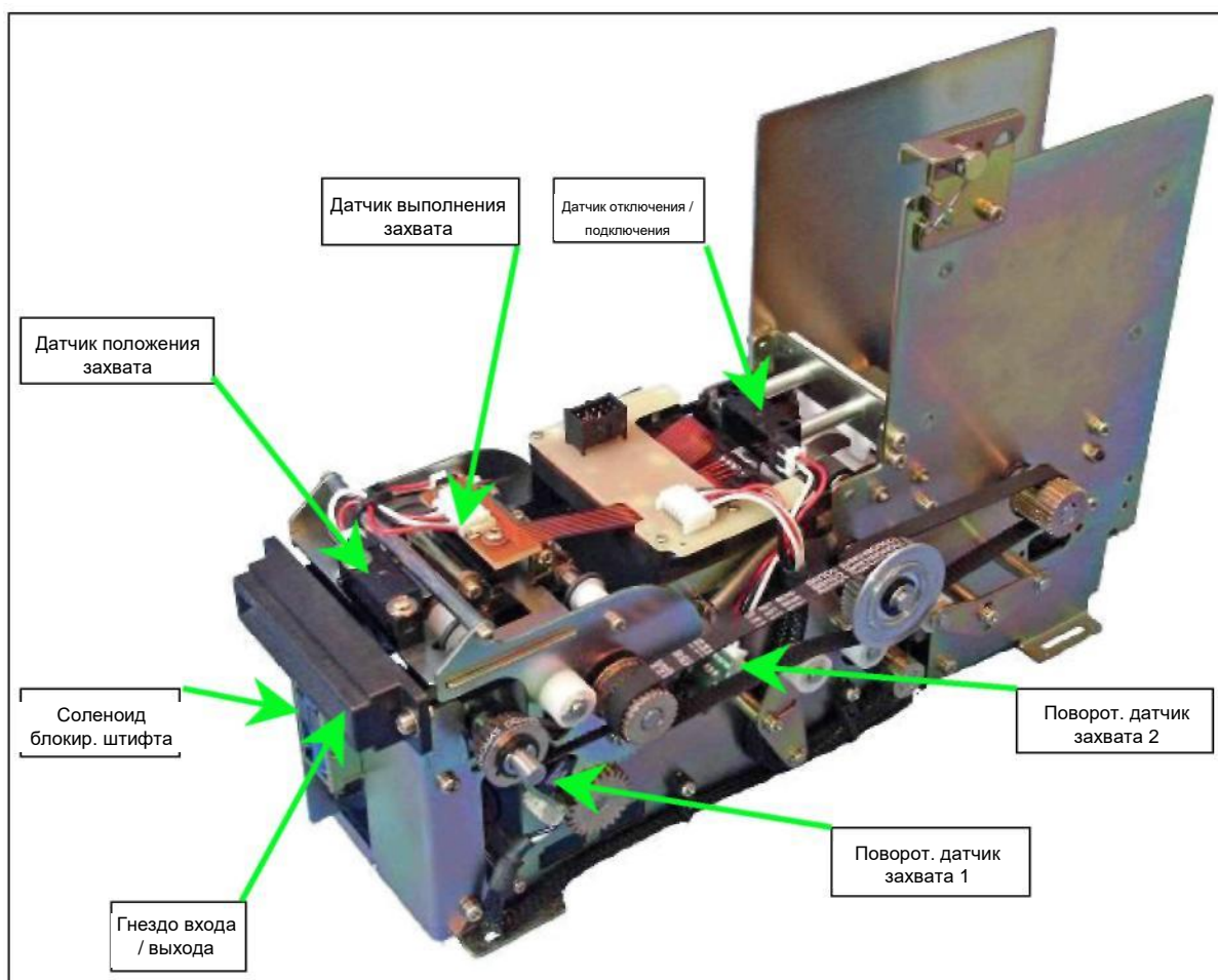
Рисунок 4 – Положение датчиков, гнезда и клапана блокировки устройства SCD-2500
