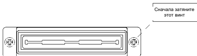
Рисунок 22 – Затягивание крепежных винтов гнезда входа/выхода
