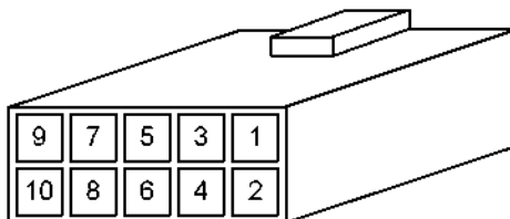
Рисунок 15: Корпус сопрягающего соединителя контактного интерфейса
