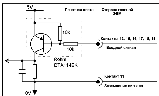
Рисунок 2 – Цепь входного сигнала
