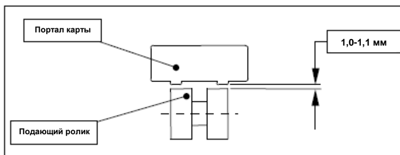
Рисунок 18 – Регулируемый зазор
