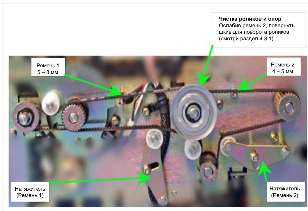
Рисунок 19 – Регулировка приводного ремня
