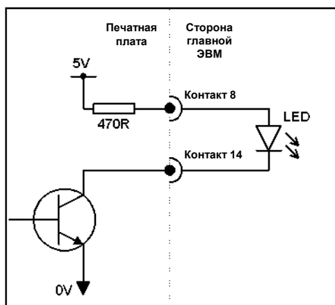
Рисунок 13 – Выходная цепь светодиода
