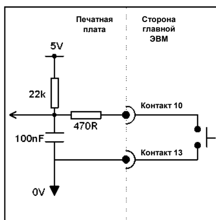
Рисунок 14 – Входной контур нажимной кнопки
